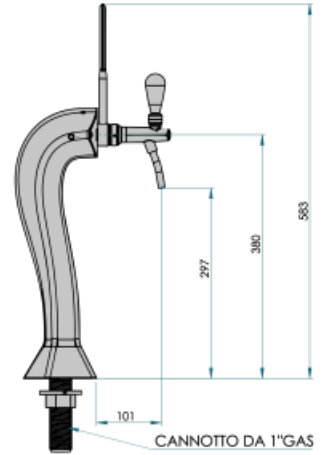
CANNOTTO DA 1" GAS
