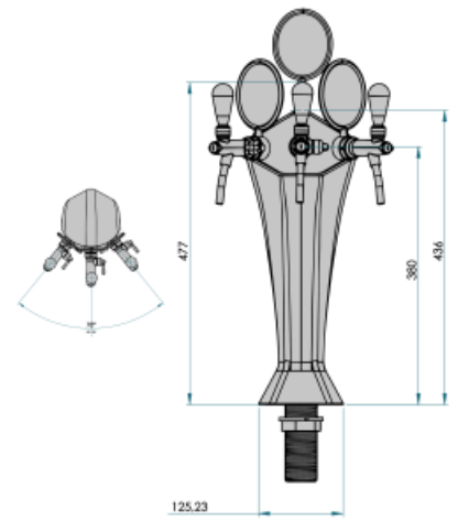
CANNOTTO DA 1" GAS
