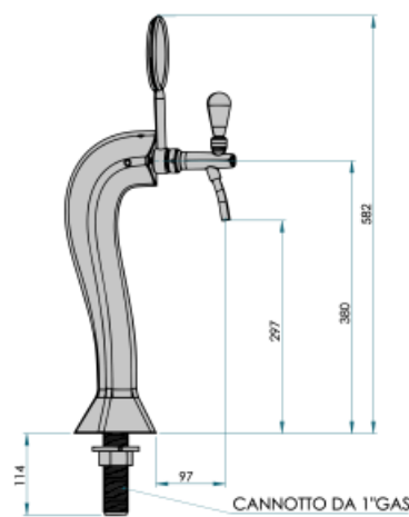
CANNOTTO DA 1" GAS
