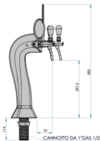
CANNOTTO DA 1" GAS 1/2
